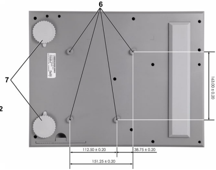
底視圖
